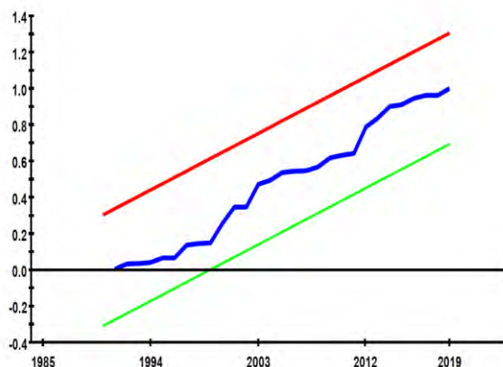
نمودار ۳. آزمون مدل خطی CUSUMSQ
