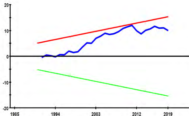
نمودار ۲. آزمون مدل خطی CUSUM
